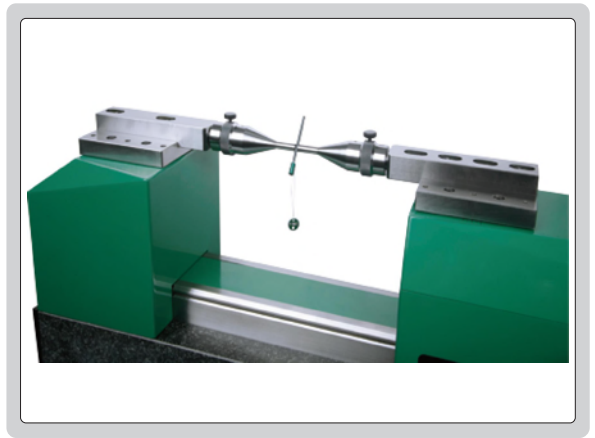
针规测量
