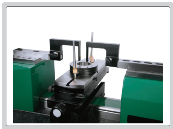
环规测量
