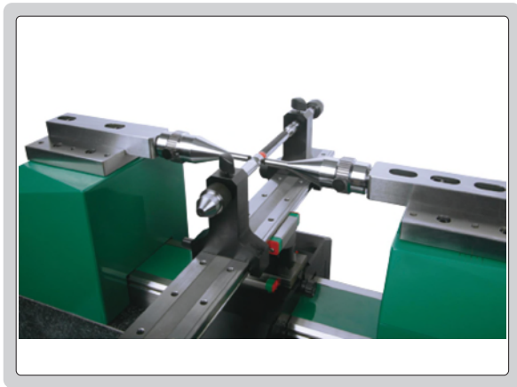
塞规测量
